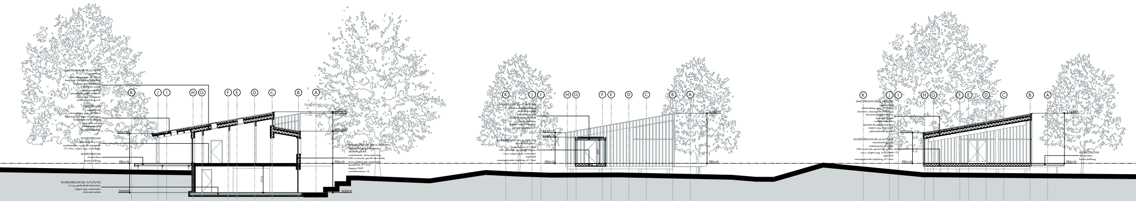
Doorsnede D-D
